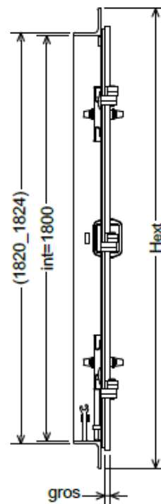
secțiune verticală
